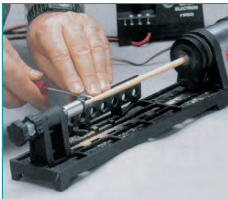
Verjüngen von Masten und Rahen mit Stechbeitel und Auflagebock. Anschließend mit Sandpapier überschleifen.
