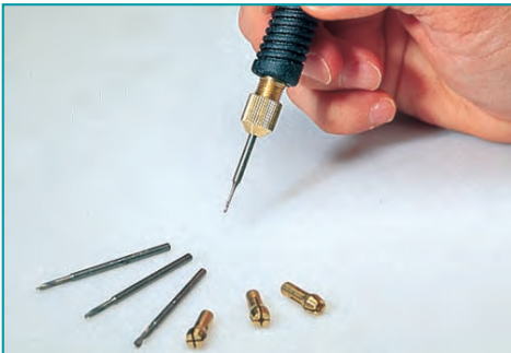
Bohren mit Bohreinsätzen für 0 - 3 mm Bohrer
