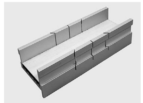
Bestell-Nr. 3135 Präzision-Schneidlade aus Aluminium mit 4 mm Opferholz Einlage, für die Micro-Handsäge 3134 und Mini-Ryoba 3094, mit Anschlagkante um die Schneidlade sicher an der Tischkante zu fixieren. Länge 137 mm, Breite 45 mm, Höhe 32 mm
