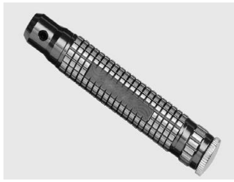
Bestell-Nr. 3083 Werkzeug-Handgriff, passend für viele Werkzeuge (z.B. Nadelfeilen, Sägeblätter usw.). Der Schlüssel zum Wechslen ist im Kopf des Griffes integriert. Durchmesser 15 mm, Länge 88 mm
