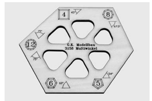
3158 Multiwinkel: Mit dem Multiwinkel lassen sich die gängige Winkel für Gehungen an Ihren Holzbearbeitungsmaschinen genau einzustellen. Dieses unregelmäßige Sechseck kann an Tischkreissägen, Hobelmaschinen, Tischfräsen, Radialsägen, Bandsägen, Tischbohrmaschinen usw. benutzt werden.
