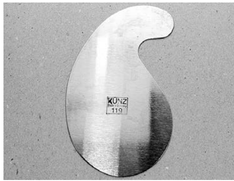
Bestell-Nr. 3148 Schwanenhalsziehklinge, Abmessung ca. 120 x 65 mm
