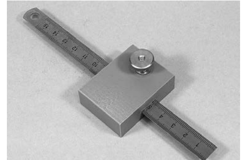
Bestell-Nr. 3174: Linealanschlag mit 150 mm Edelstahllineal und justierbarem ABS-Anschlag.
