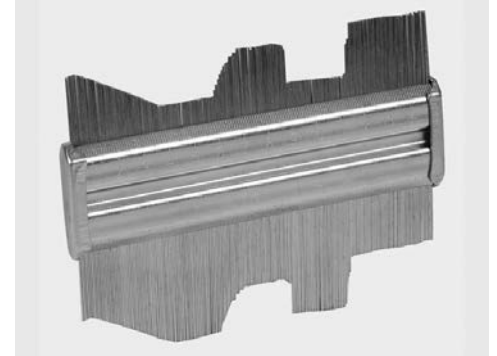
Bestell-Nr. 3089 Stahl-Formlehre, feine Stahlstifte erlauben akurates Übertragen und Vervielfältigen von irregulären Formen, Maximale Profiltiefe 45 mm, Profillänge 150 mm
