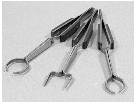
Bestell-Nr: 3154 Selbstschließende Lötpinzetten, 3er Satz je eine für runde, ovale und eckige Werkstücke, aus rostfreier Stahl mit Wärmeschutz, Länge ca. 160 mm
