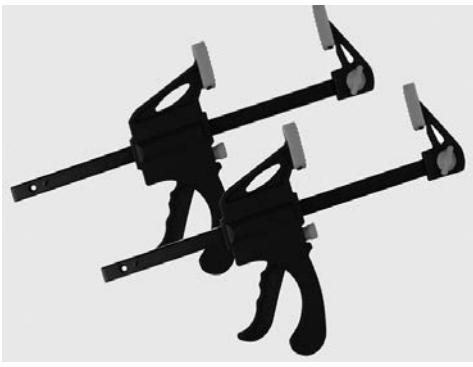
Bestell-Nr. 3081 2 Einhand-Schnellspannzwingen, Spannweite 100 mm, Spreizweite 130 mm
