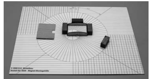
Bestell-Nr. 3029 „Magnet Montagehilfe“ (20 x 25 cm) Zum Lieferumfang gehören 4 starke Magneten 10 x 10 x 25 mm, diese dienen als Anschlag.
